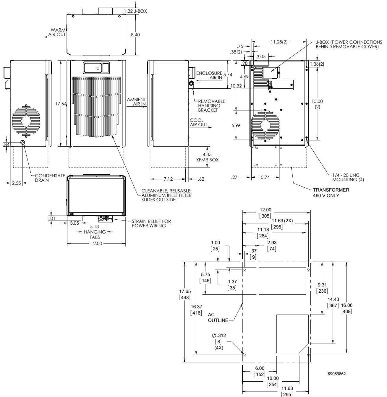
Cutout Dimensions
